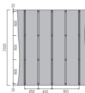
Toepassing regelwerk 450 mm met rozetten en schroeven voor BA 12,5 mm.
