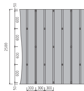
Toepassing regelwerk 300 mm met rozetten en schroeven voor BA 12,5 mm.
