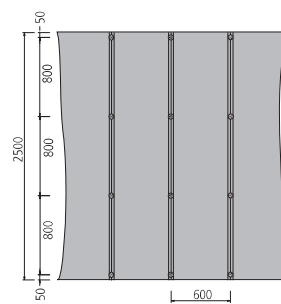
Toepassing regelwerk 600 mm met rozetten en schroeven vanaf BA 20 mm.
