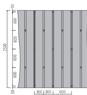
Toepassing regelwerk 300 mm met rozetten en schroeven voor BA 10; BA 12,5 mm.
