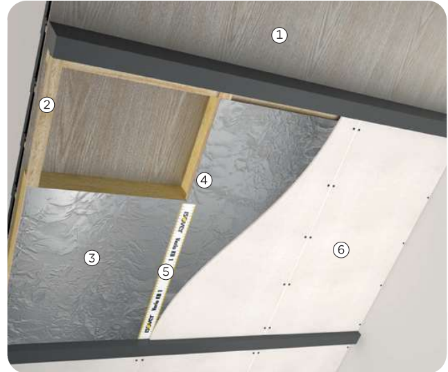
Figuur 3: verwerking Isover Rollisol Plus tegen verticale latten
