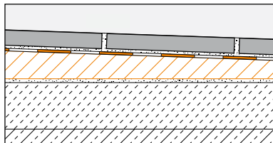
Schlüter®-KERDI-SHOWER op nivelleringsdekvloer
