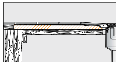
Inbouwvoorbeeld Schlüter®-KERDI-SHOWER-TT
