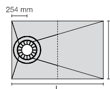
Schlüter®-KERDI-SHOWER op nivelleringsdekvloer
