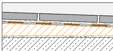
Schlüter®-KERDI-SHOWER-T
