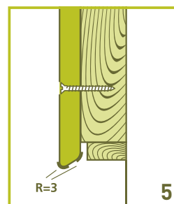
Afronden. Niet recht afschuinen.
