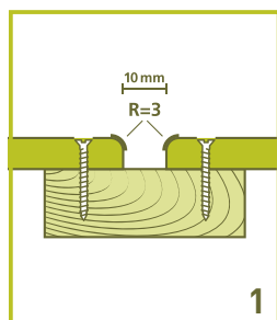
Open voegen. Geen stuiknaden.
