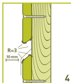
Waterslagprofiel. Geen H-profiel.
