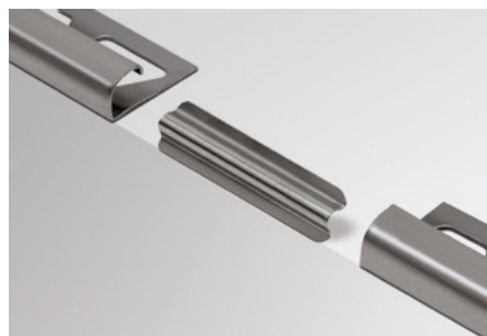
Schlüter®-RONDEC-E/V (verbindingstuk voor roestvaststalen profielen)
