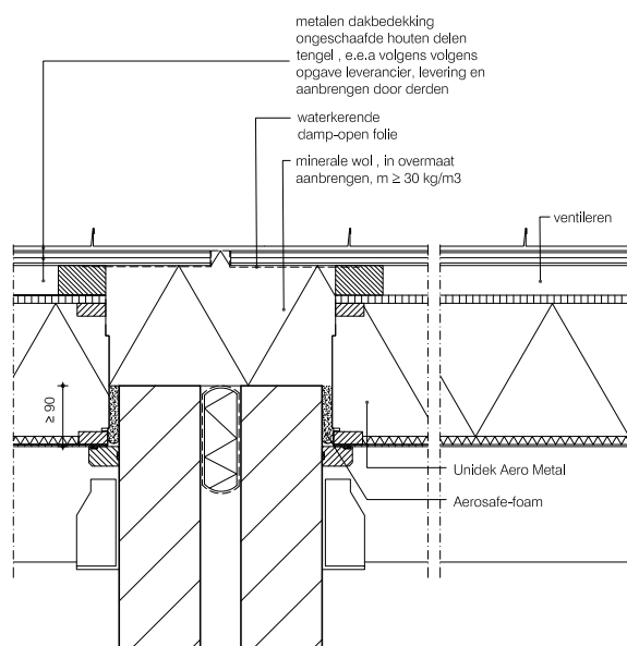
Detailtekening 1 - Woningscheidende wand Unidek Aero Metal geventileerd
