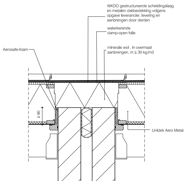
Detailtekening 2 - Woningscheidende wand Unidek Aero Metal ongeventileerd
