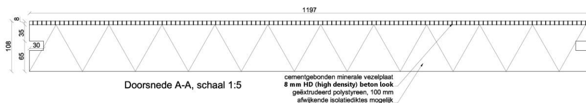
CEBO geïsoleerde kantplank l tot = 1197 mm
