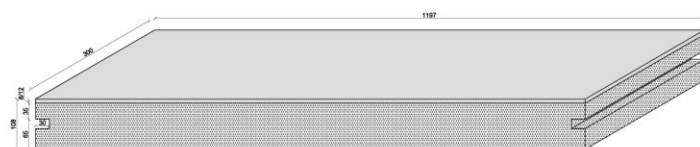
CEBO geïsoleerde kantplank l tot = 1197 mm
