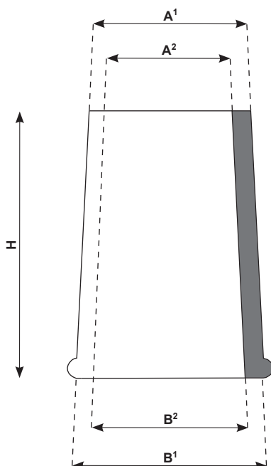
Doorsnede schoorsteenpot taps
