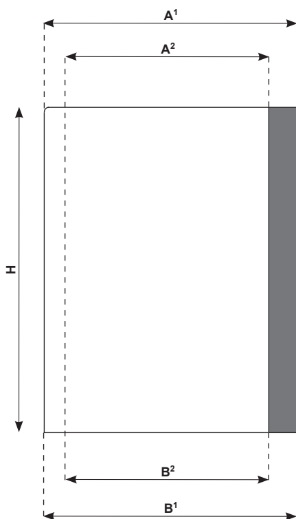
Doorsnede schoorsteenpot recht
