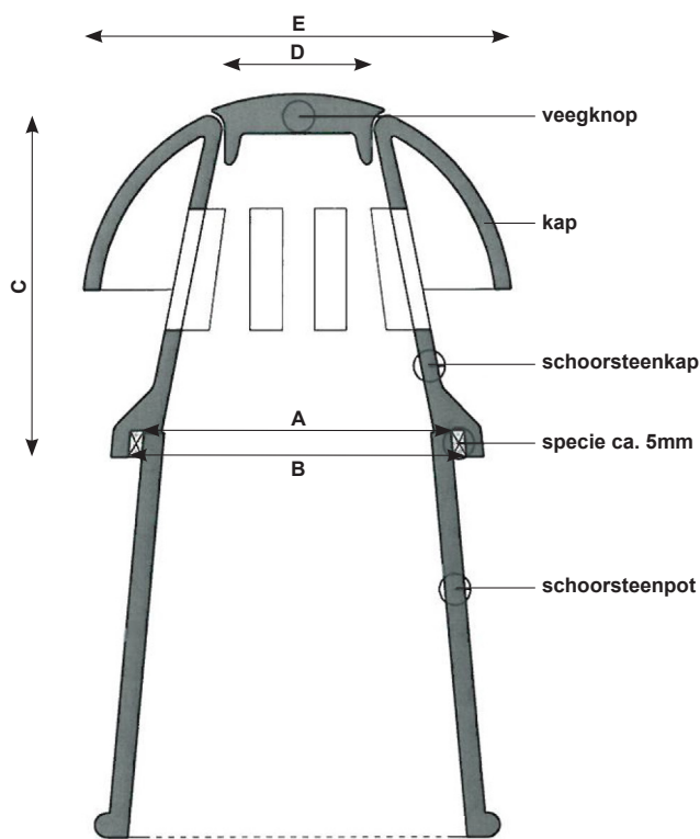
Doorsnede schoorsteenkap
