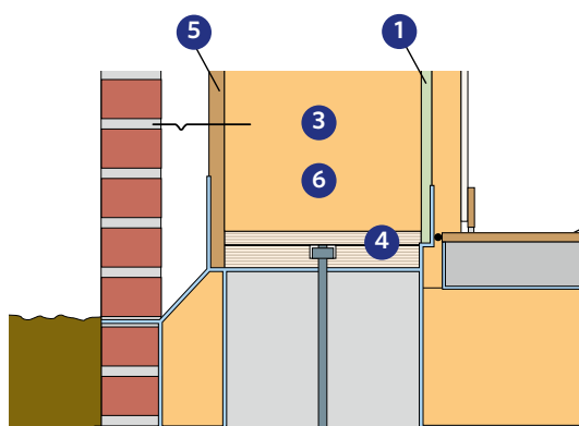
Funderingsaansluiting
