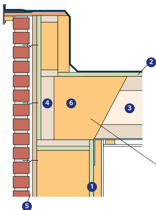
Wand met platdak aansluiting
