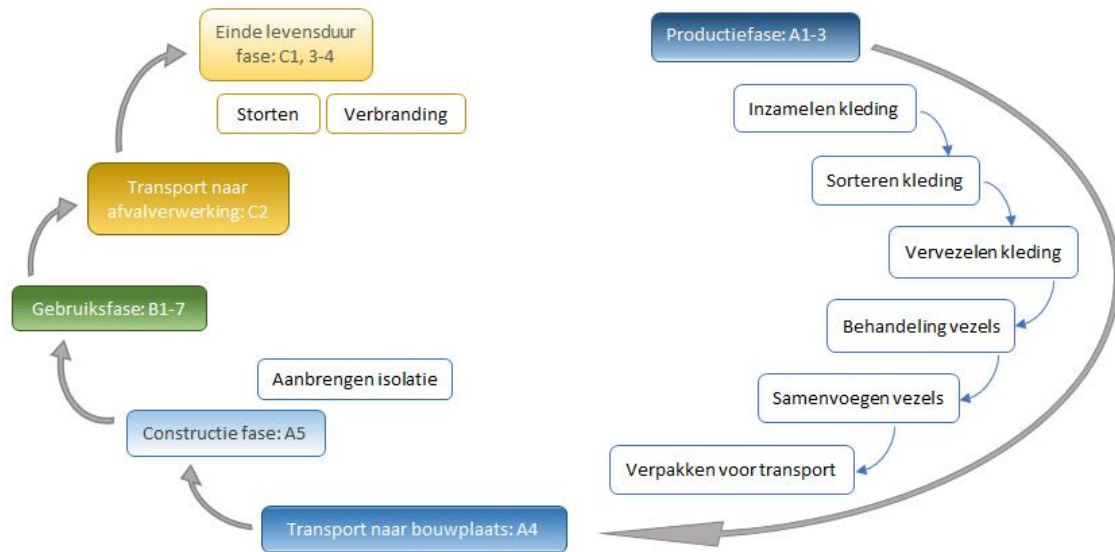
Figuur 2: Flowchart Métisse® katoen isolatie
