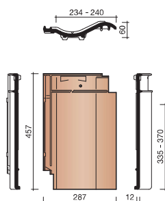
0000 MADURA DAKPAN
