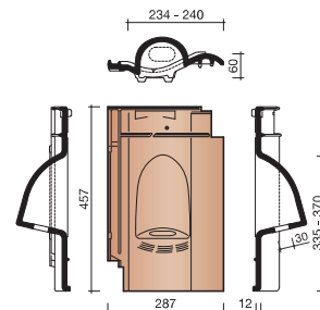
8660 GIERZWALUWPAN
