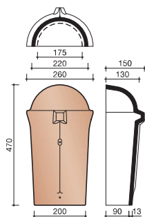
3110 BEGINSCHUBVORST
