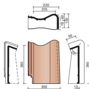
7590 RECHTER GEVELCHAPERONPAN
