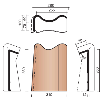
7580 LINKER GEVELCHAPERONPAN
