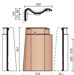
7080 LINKER GEVELPAN
