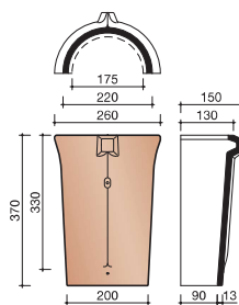
3100 SCHUBVORST
