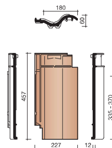
8030 DRIEKWART PAN
