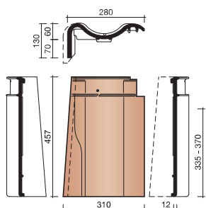
8545 GEVELAANSLUITPAN LINKS
