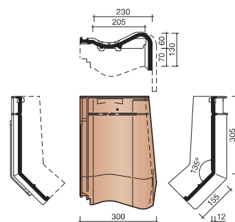
7290 RECHTER GEVELKNIKPAN
