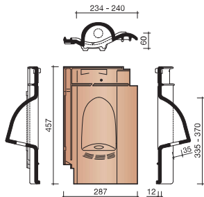
8655 MUSSENPAN
