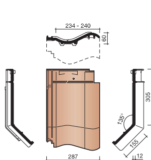
8200 KNIKPAN
