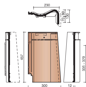
7090 RECHTER GEVELPAN
