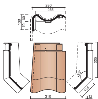
7280 LINKER GEVELKNIKPAN
